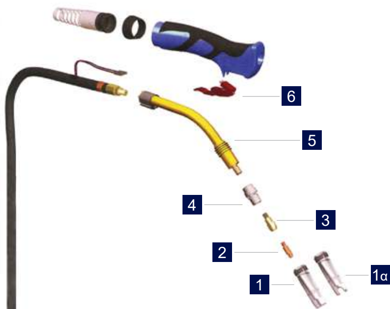
ΤΣΙΜΠΙΔΕΣ ERGOPLUS 36
